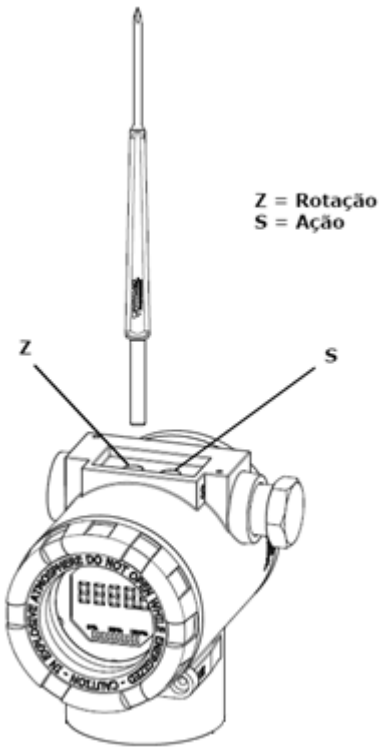
Figura 3.1 – Z e S do ajuste local e chave magnética.
