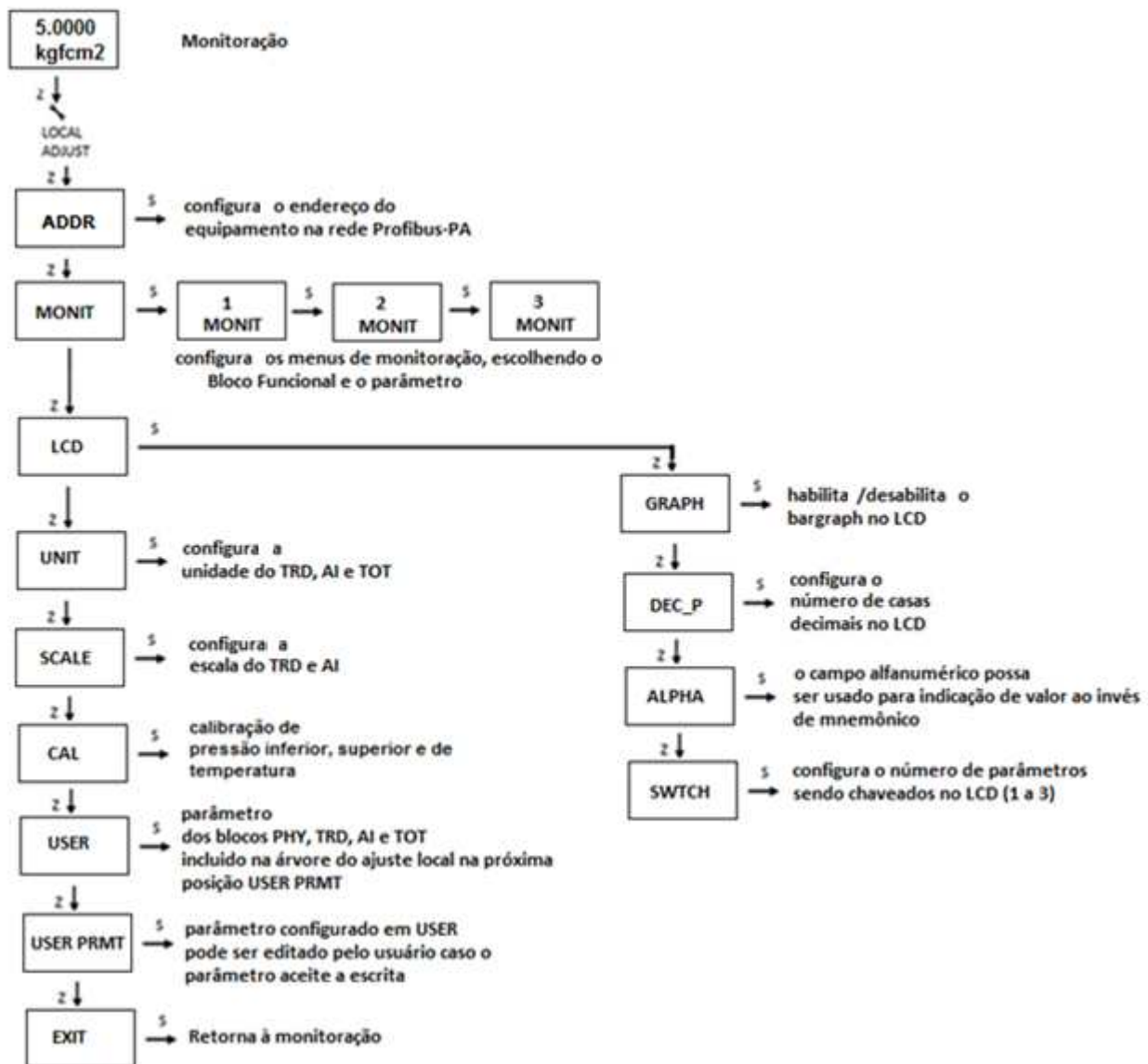
Figura 3.5 – Árvore de programação do ajuste local do VPT11-P.
