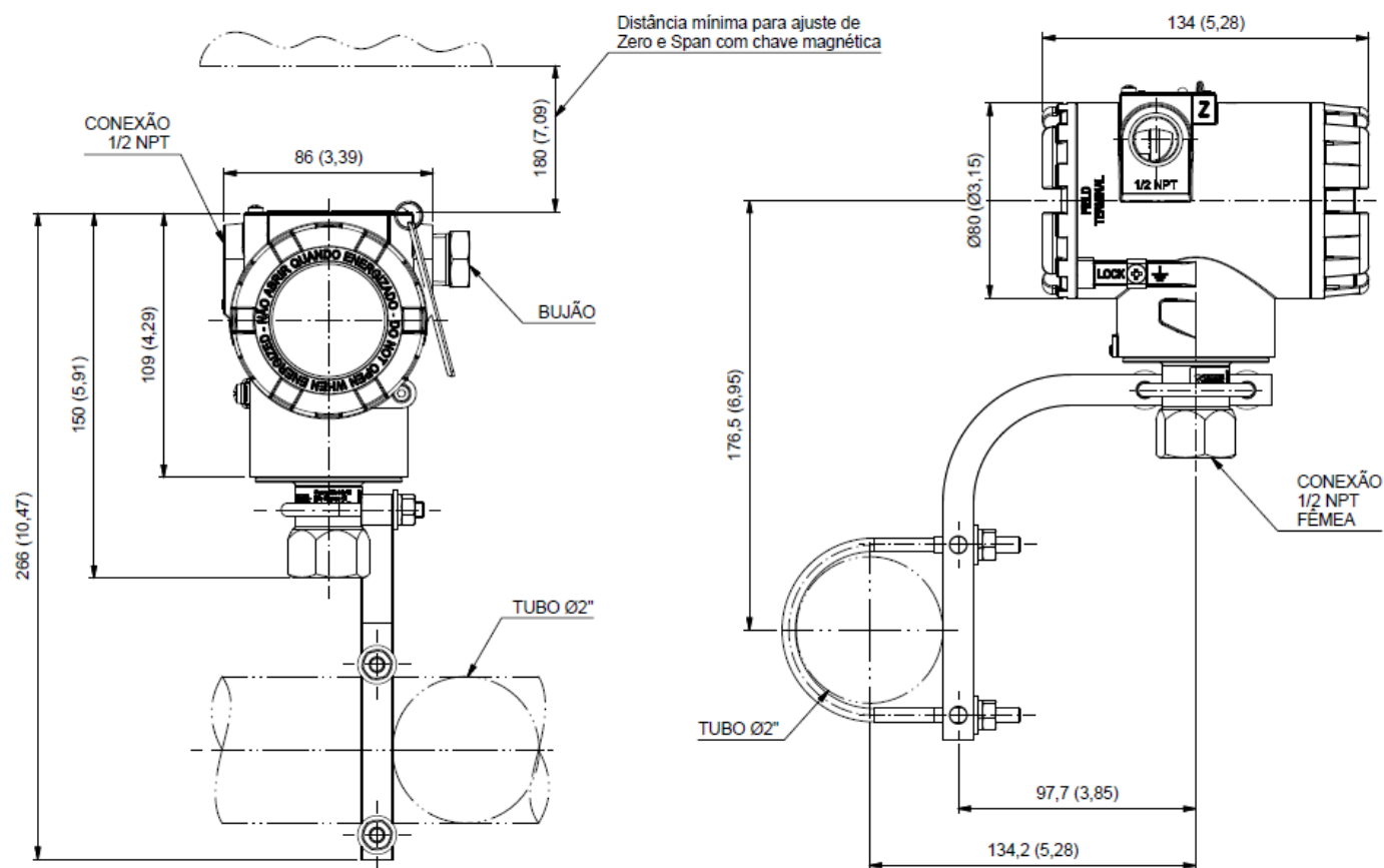
Figura 2.1 – Desenho dimensional e esquema de montagem do VPT11-P.
