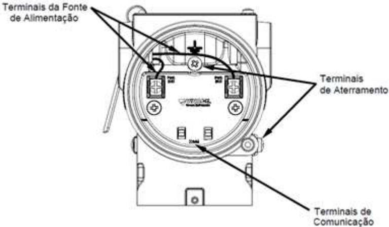
Figura 2.7 – Conexões e descrição dos terminais do VPT11-P. Tabela 2.2 – Descrição dos terminais do VPT11-P.
