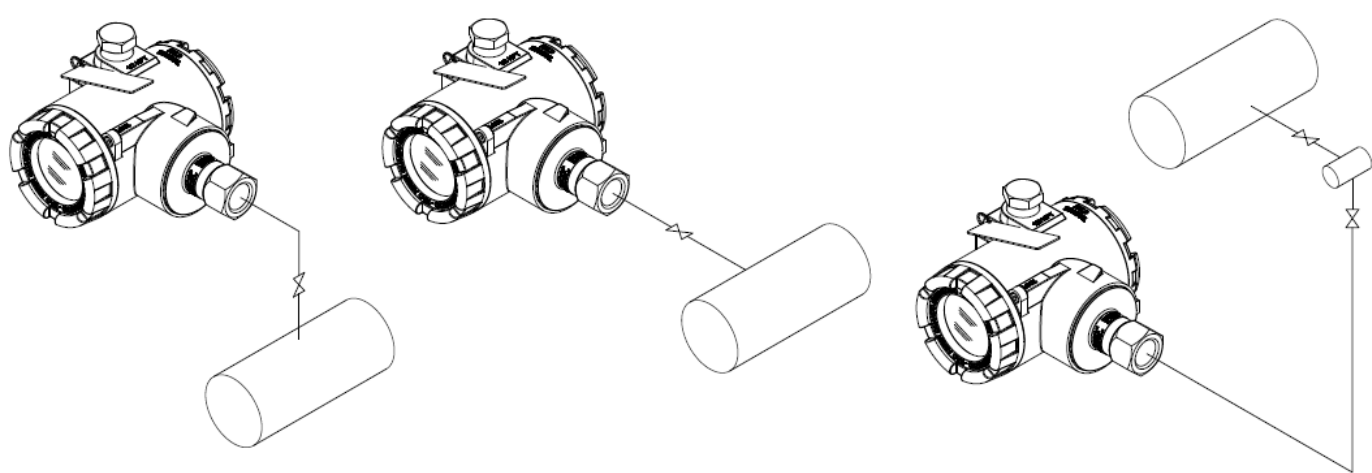
Figura 2.5 – Exemplos de montagem do transmissor, em relação à tomada de pressão.
