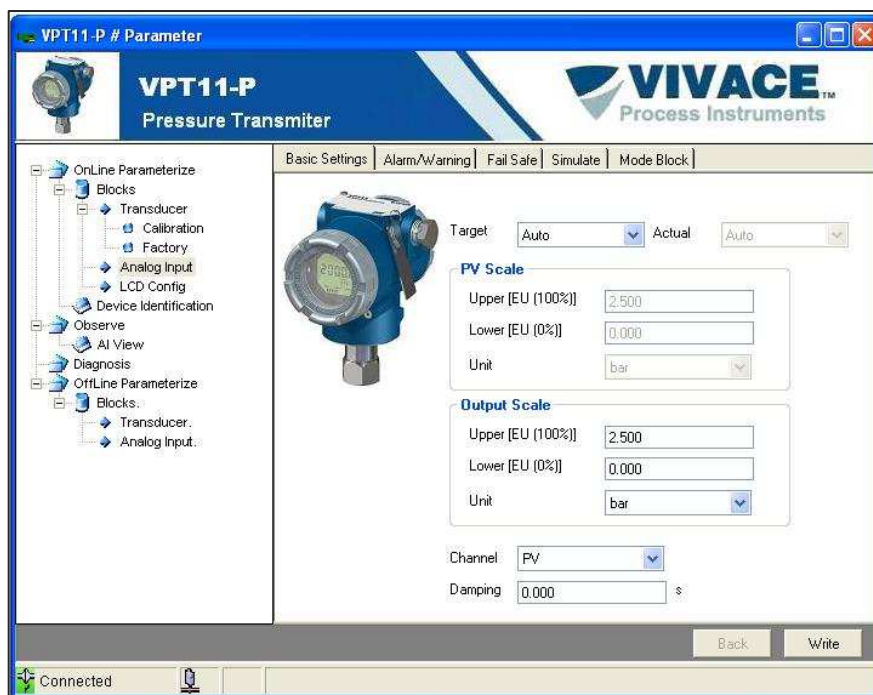
Figura 3.8 – Tela de configuração do VPT11-P no PACTware.
